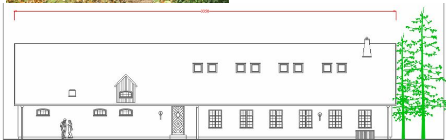
Fasad mot öster Sk 1:100
